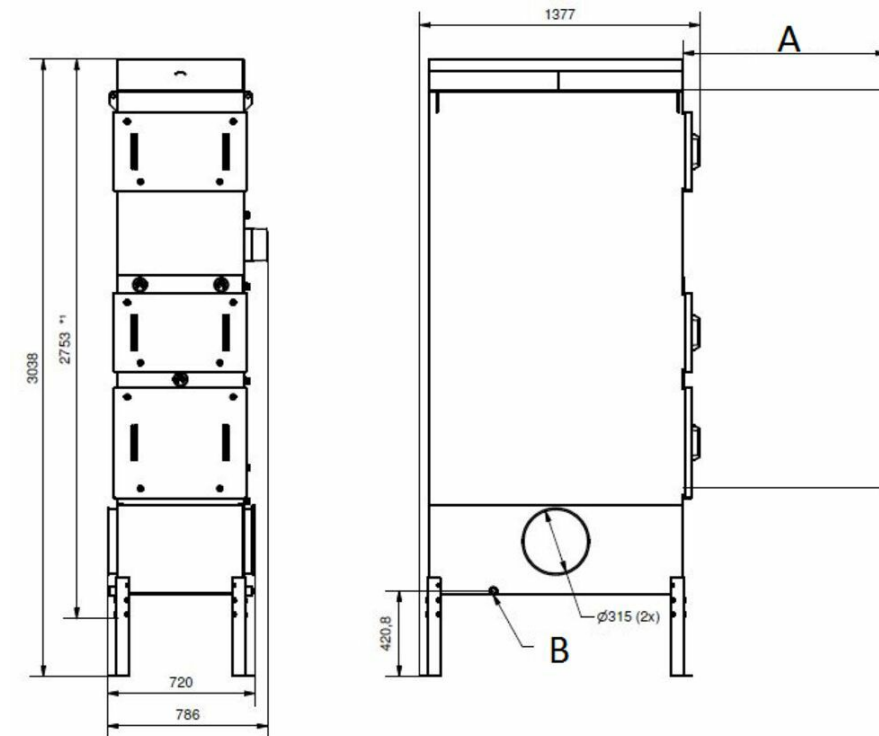
A) 1000 mm plads for filter service B) Drænstuds (x2)
